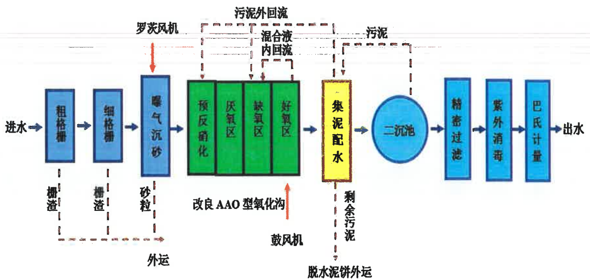
图 5-1 三灶厂环保设施运行流程图
